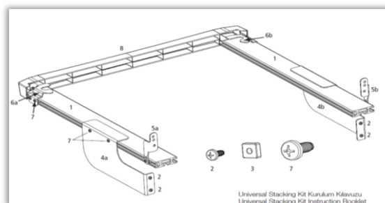
NÁKRES kovového mezikusu
