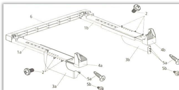
NÁKRES plastového mezikusu
